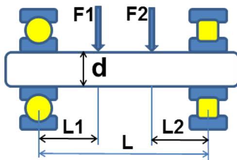
図 3 軸受の寿命計算
